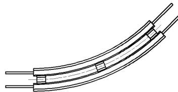
Horizontale Gleitbögen
